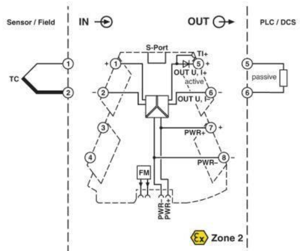
MINI MCR-2-TC-UI
