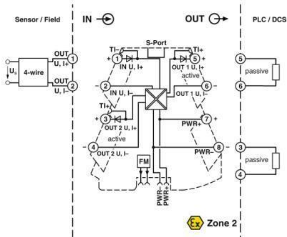
MINI MCR-2-UNI-UI-2UI
