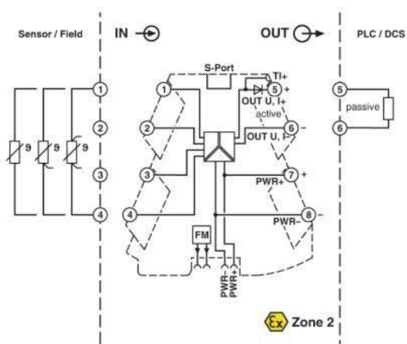
MINI MCR-2-RTD-UI
