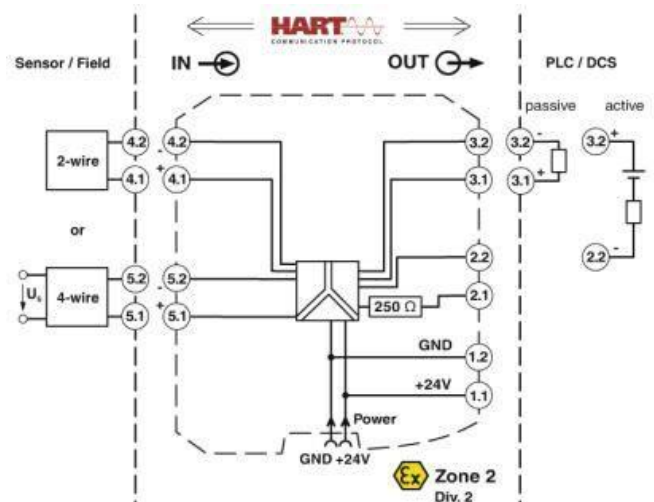
MACX MCR-SL-RPSSI-I
