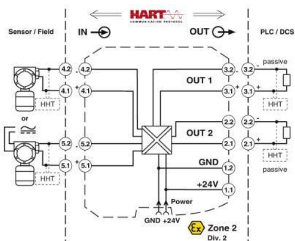
MACX MCR-SL-RPSSI-2I
