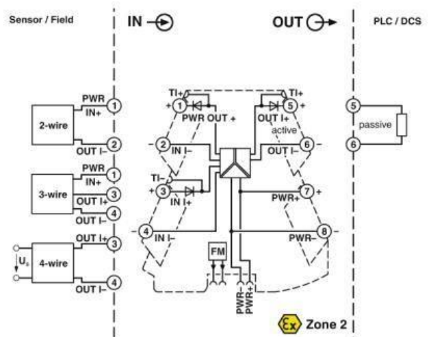
MINI MCR-2-RPSS-I-I
