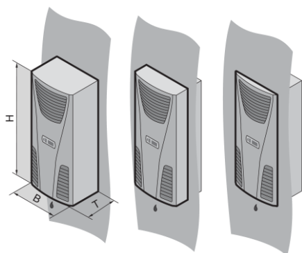
รูปแสดงการติดตั้งได้ 3 แบบ
