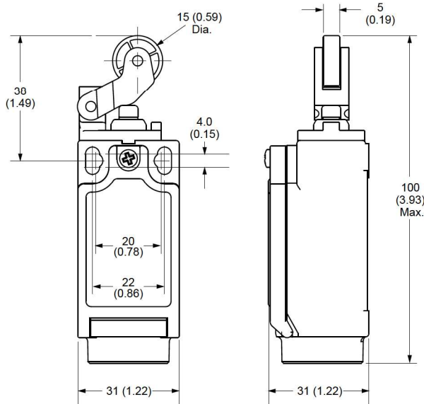
Hinge Lever
